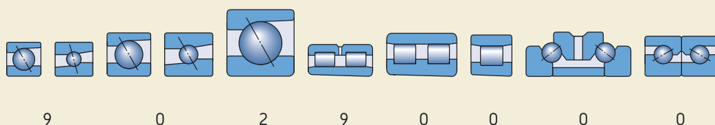
精密主轴轴承的直径系列
